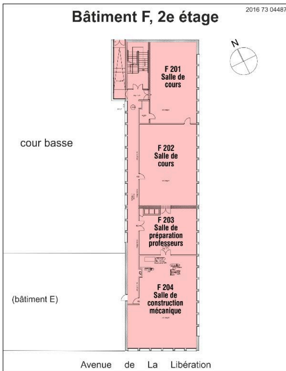
Bâtiment F, 2e étage, plan de localisation des machines
