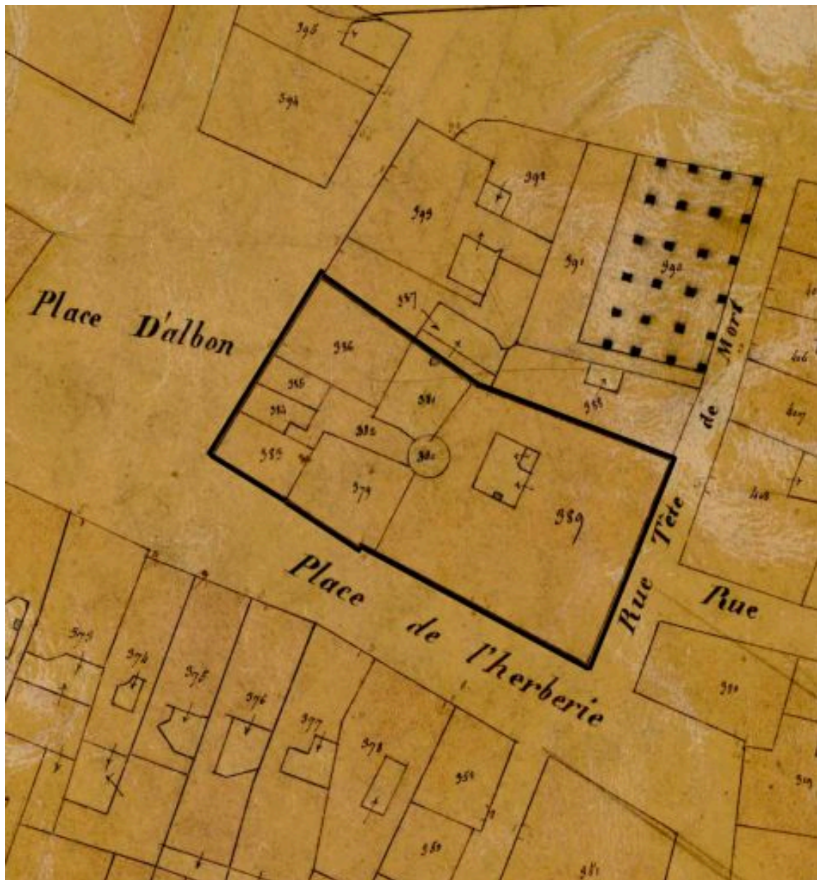
Plan-masse, extrait du plan cadastral levé en 1831, section F
