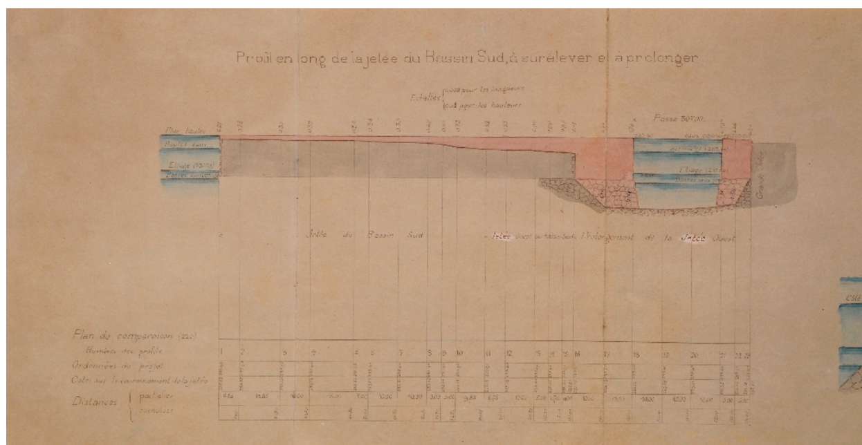
Exhaussement du bassin sud, coupe longitudinale, 1904
