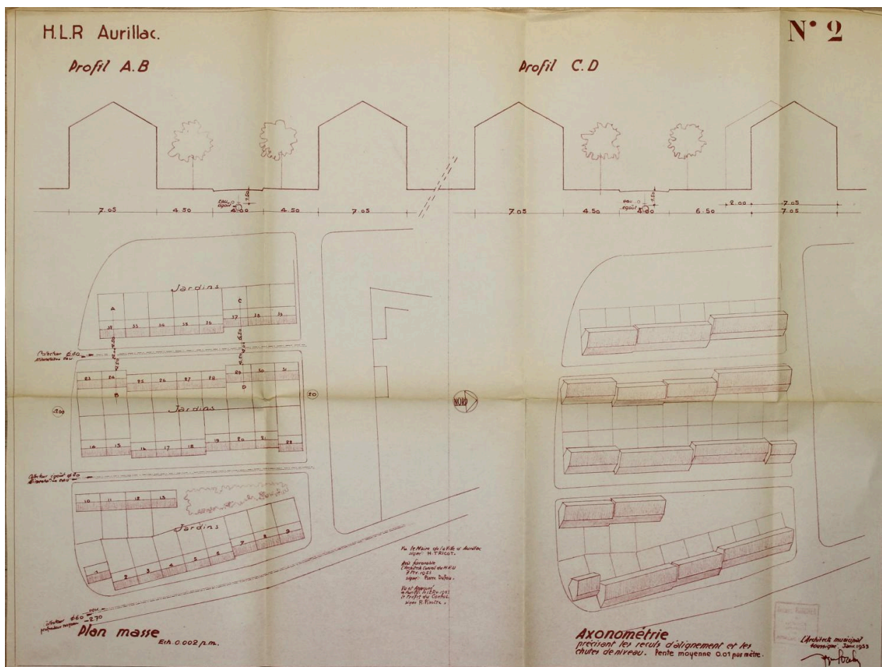
Aurillac, cité des Camisières, plan-masse, profils et axonométrie du 1er programme de maisons HLR, janvier 1953, Jacques Porcher architecte (Archives municipales d'Aurillac, 135 W 34, permis de construire n° 1267).
