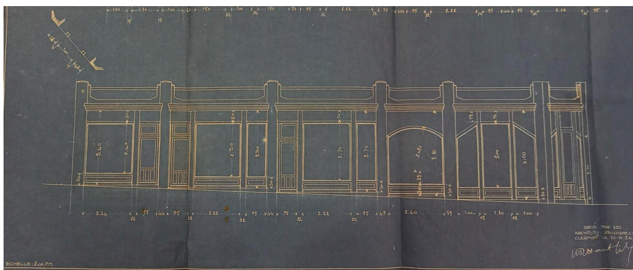
Elévation des menuiseries de devanture sur l'avenue Charras
