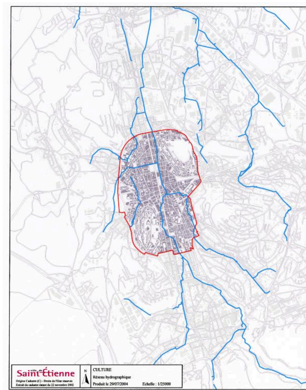
Plan du réseau des eaux, sur fond cadastral.
