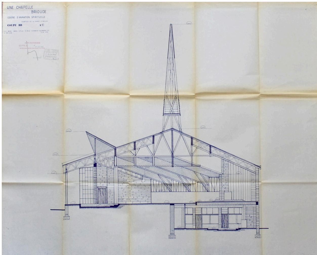
Brioude, chapelle de la Borie Darles, coupe BB (projet non définitif), 30 mars 1965, Guy Bion architecte, Archives de la paroisse Saint-Julien de Brioude.
