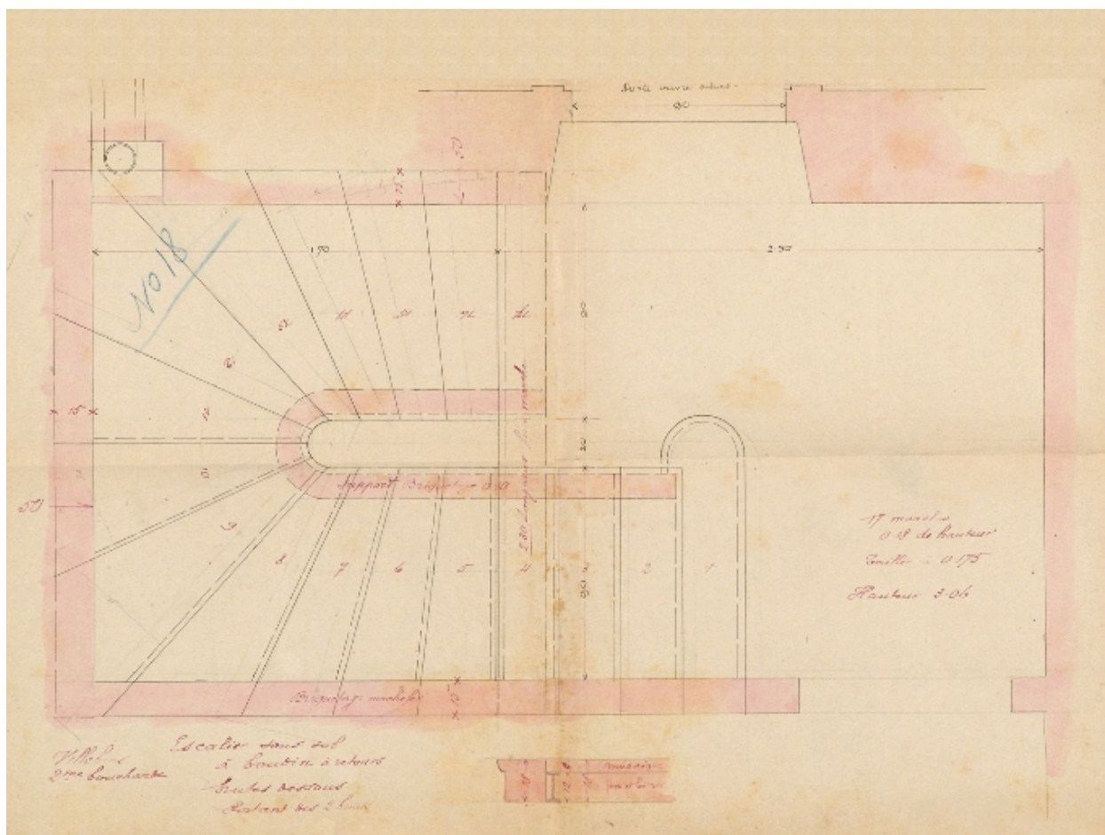
Plan de l'escalier du sous-sol
