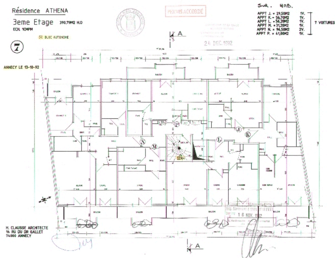
Plan du troisième étage
