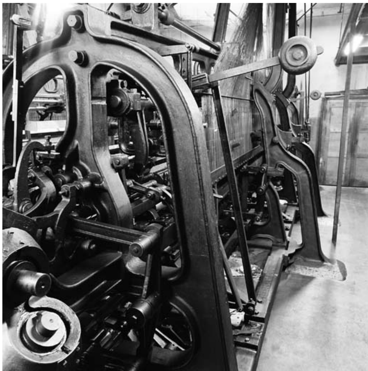
Vue arrière du métier Johnson
