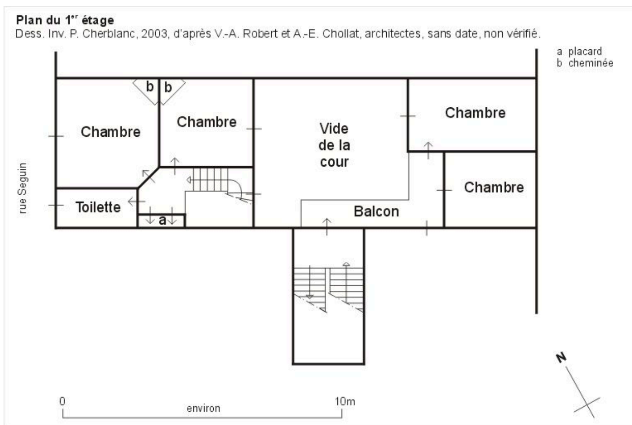
Plan de l'étage, d'après V.-A. Robert et A.-E. Chollat
