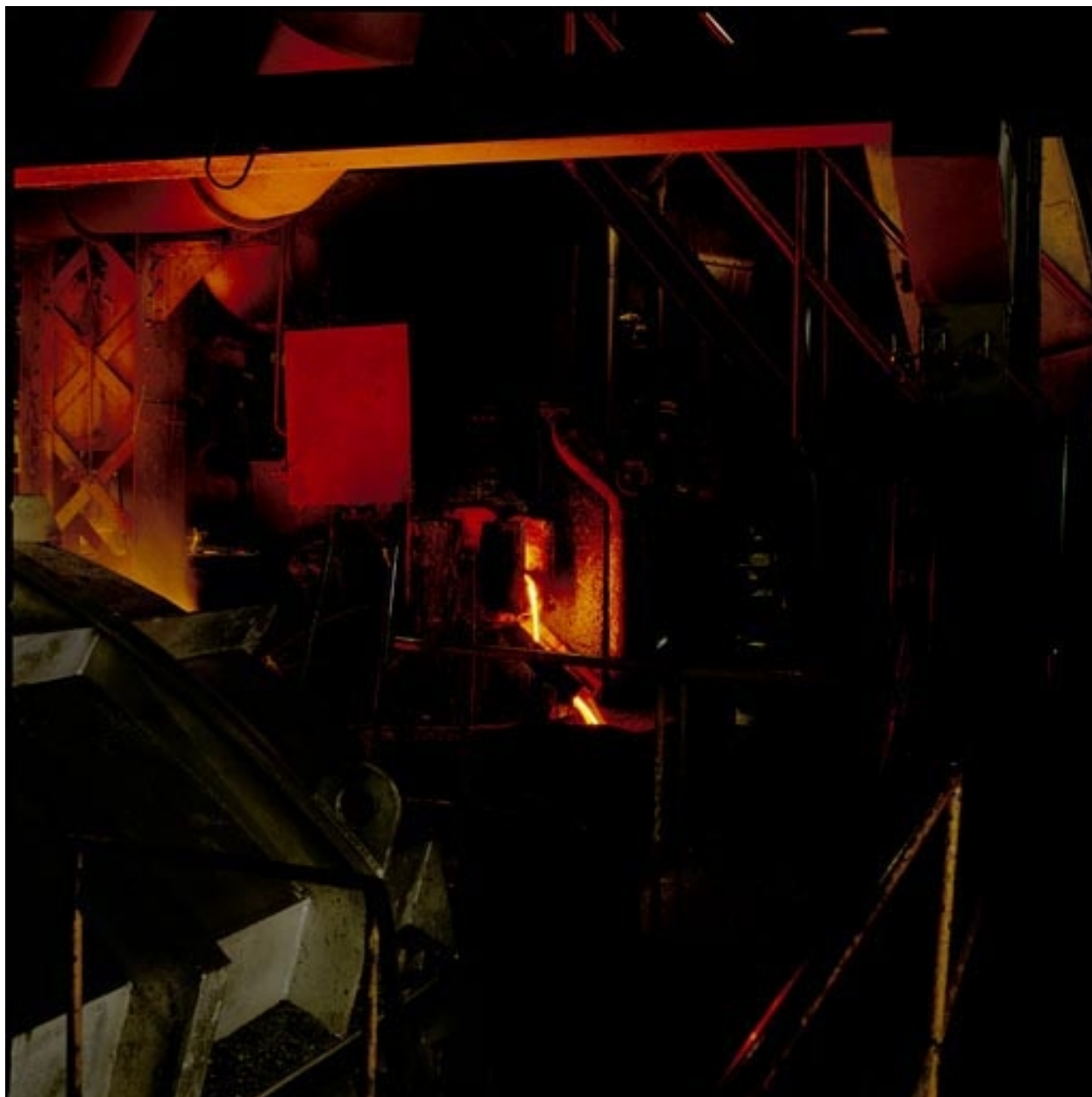
Fonderie : cubilot coulée de fonte dans le four de maintien.
