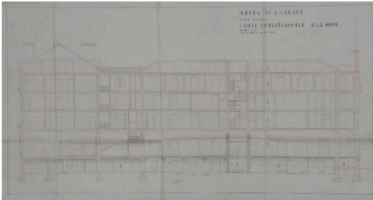
Coupe longitudinale aile nord, 1954
