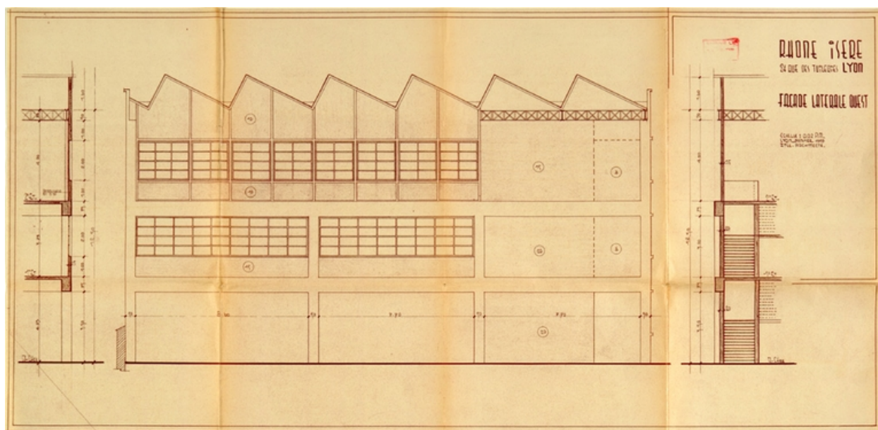
Façade latérale ouest du grand atelier
