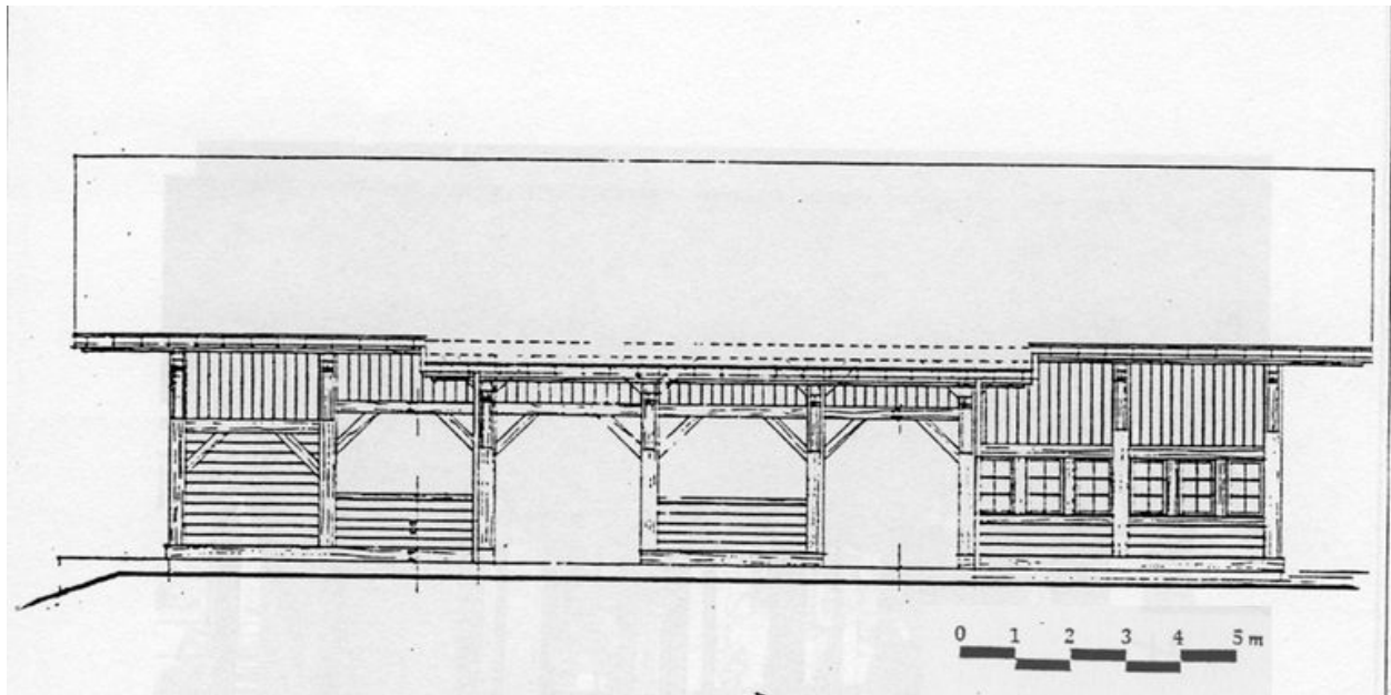
Téléphérique de Rocharbois. Élévation principale de la gare inférieure / [Pierre Duclos, 1985]
