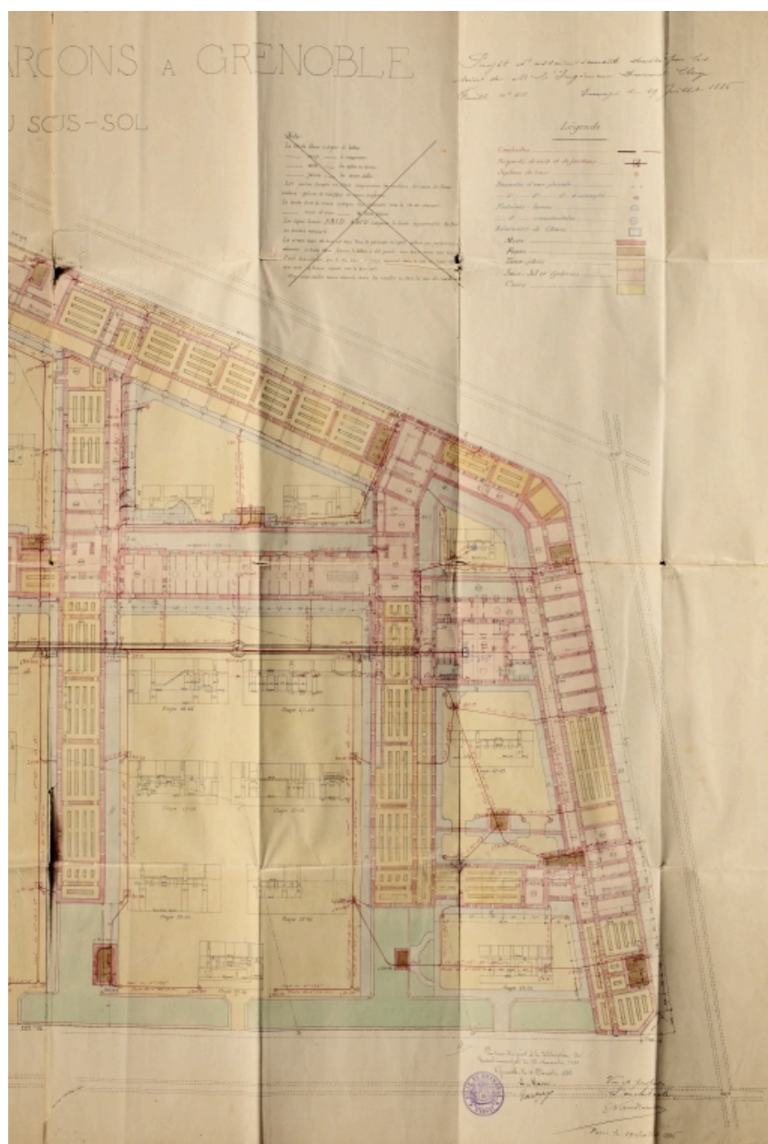
Plan du sous-sol. Détail partie droite. Document figuré. Plan. Papier. Echelle 0,0005 p.m, 41 x 60 cm. Archives municipales, Grenoble. 2 Fi 298
