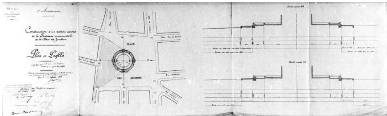
Construction d'un trottoir autour de la fontaine monumentale de la place des Jacobins. Plans et profils. 12 octobre 1887. f. pap. toile d'architecte AM Lyon. 1 S 176
