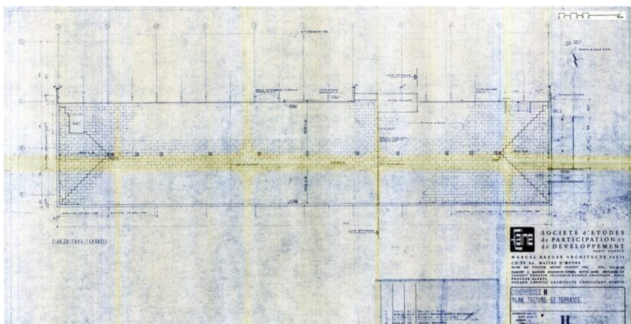
Commerces H. Plan du toit-terrasse. Marcel Breuer architecte, 29 novembre 1967 (AC Arâches-la-Frasse)
