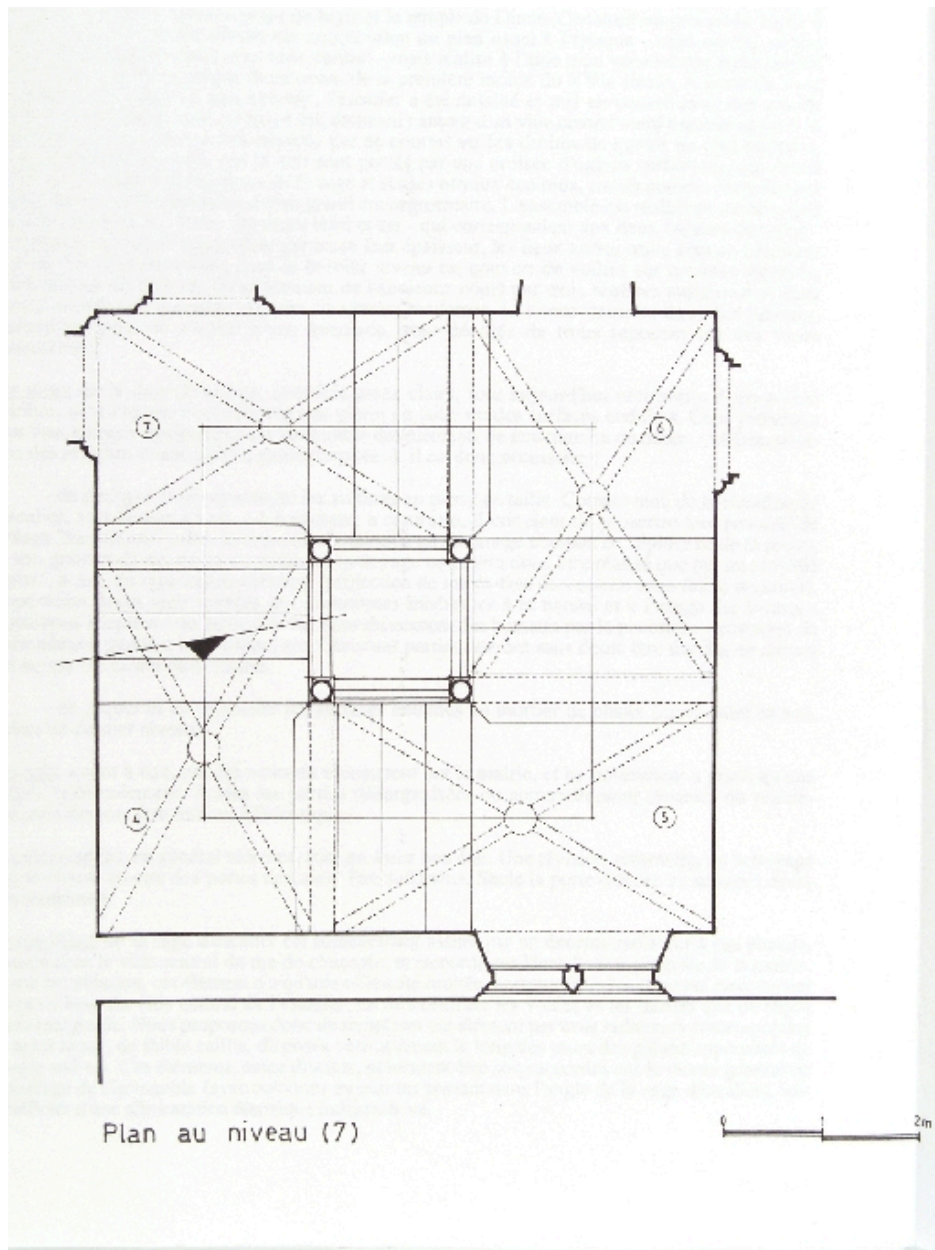
Plan de l'escalier, niveau 7
