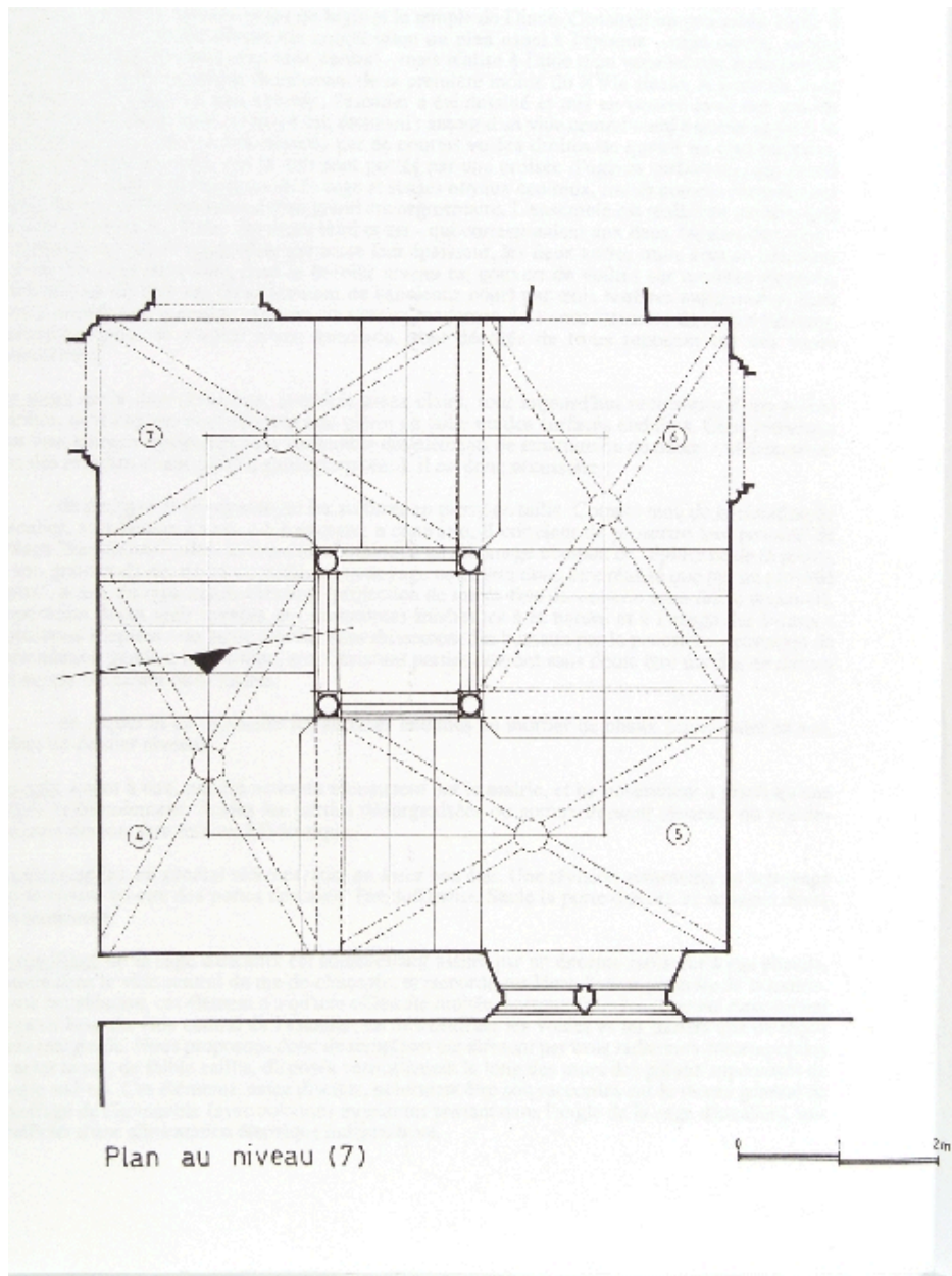
Plan de l'escalier, niveau 7
