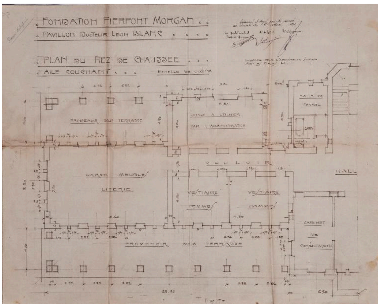
Aile ouest, 1912 : plan du rez-de-chaussée
