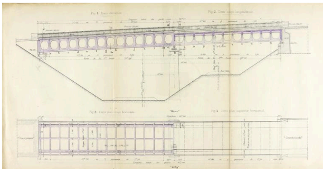
Plan et élévation du pont routier de Randan, vers 1919.
