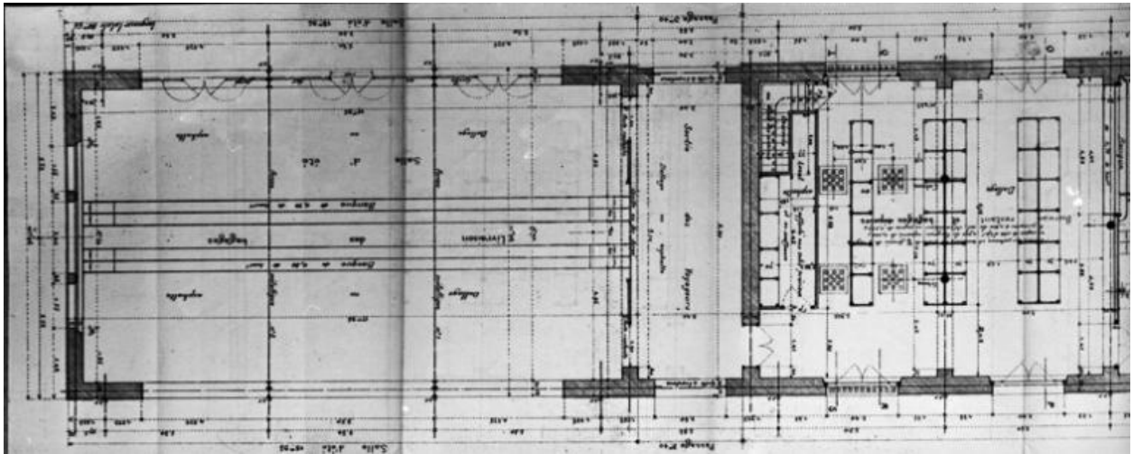
Gare de Châtel-Guyon. Bâtiment des voyageurs. Plan du rez-de-chaussée.
