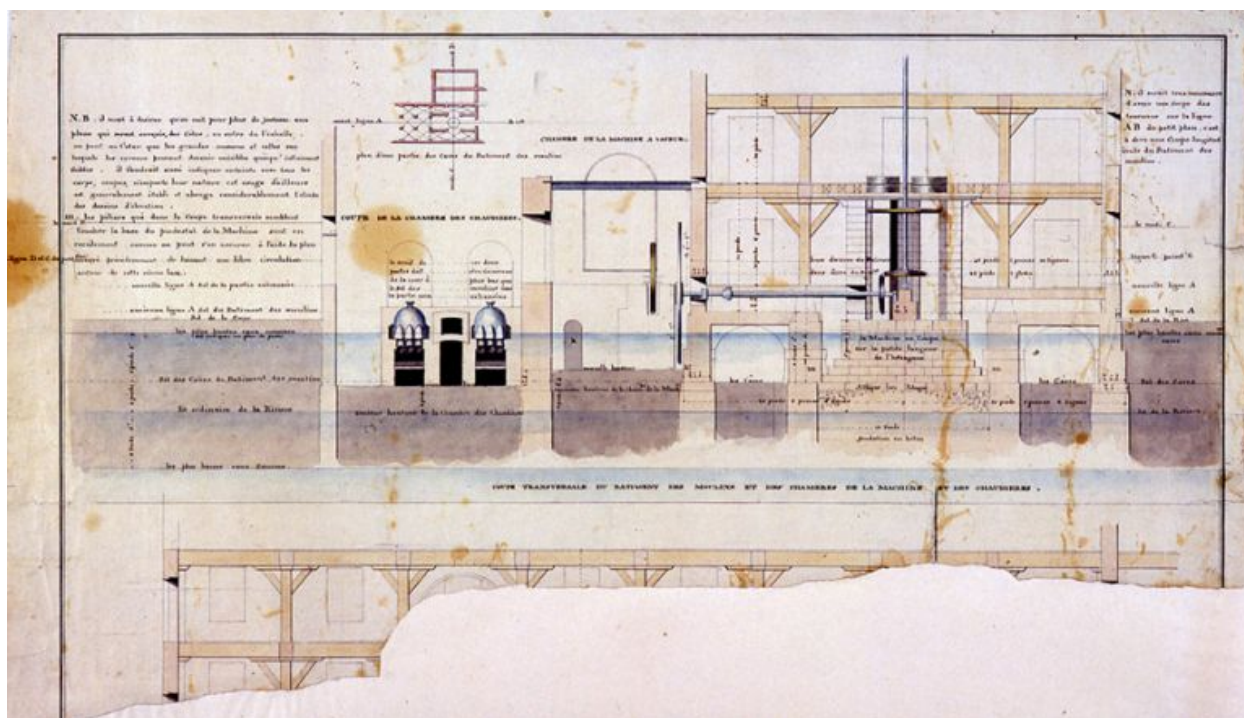
Plan de détail, coupe partielle
