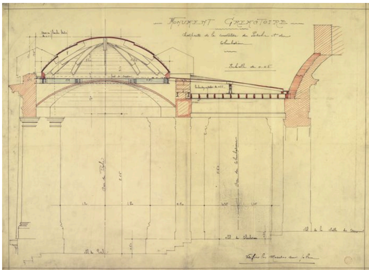
Charpente du porche et du columbarium : coupe
