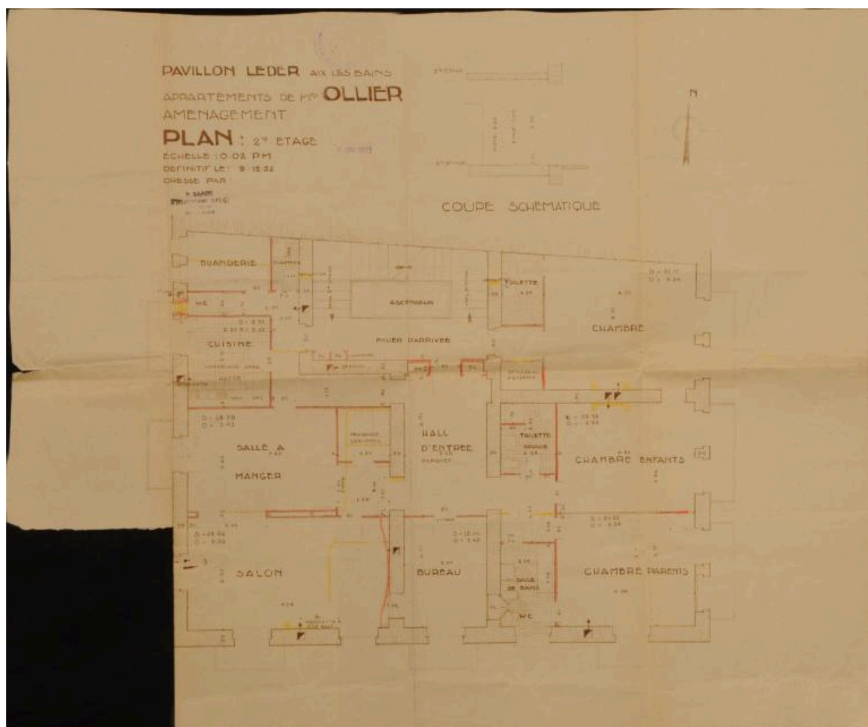
Aménagement appartement Ollier, plan 2e étage, 1952
