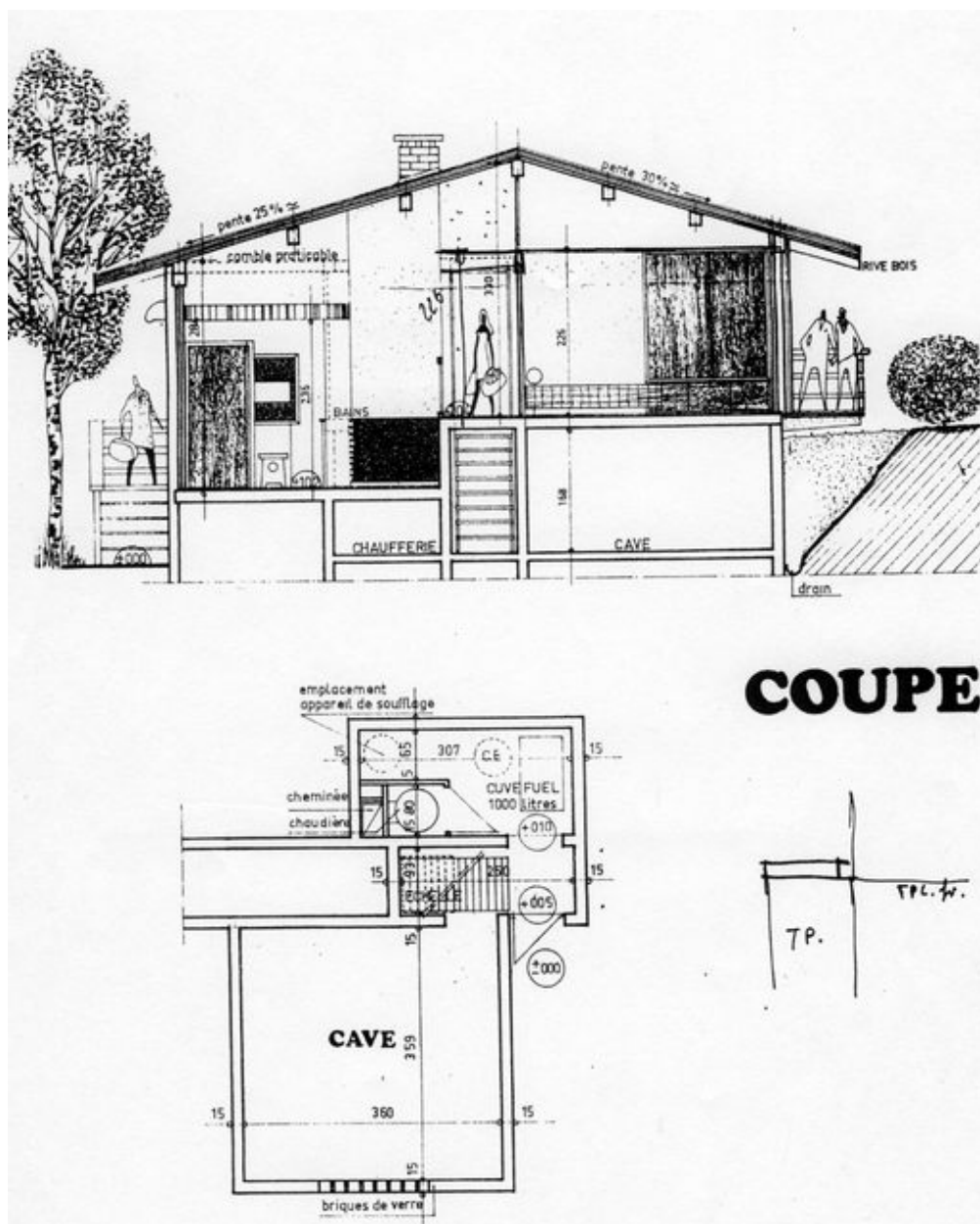
Coupe et plan du sous-sol / Georges Candilis, 1951
