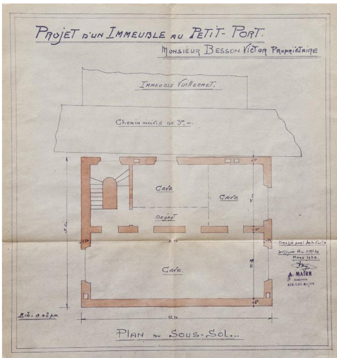
Hôtel Besson, 1934 : plan du sous-sol
