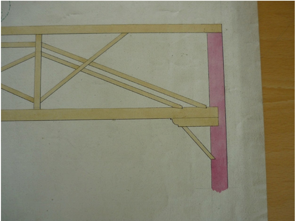
Elévation d'une charpente, s.d. (détail de la partie droite). Plan AC Lyon. Fonds des HCL ; 2OP686
