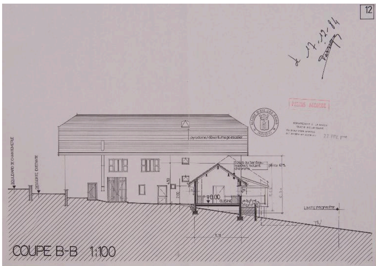
Coupe sur élévation nord, 1984
