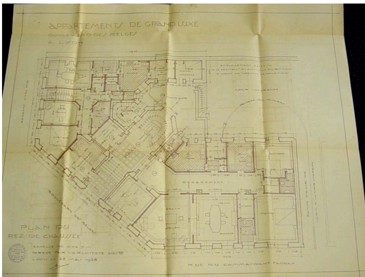
Plan du rez-de-chaussée / Bornarel, 1928
