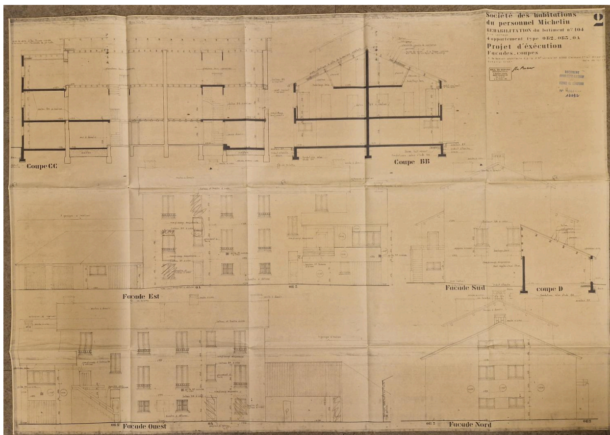
Projet de réhabilitation d'une maison de type O à Lachaux : coupes et élévations, 1979.
