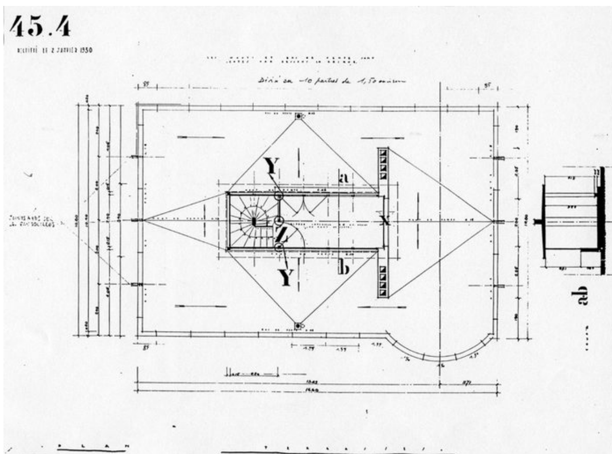
Plan du toit terrasse. Henry Jacques Le Même, Rectifié le 2 janvier 1930 (AD Haute-Savoie. 142J 574)
