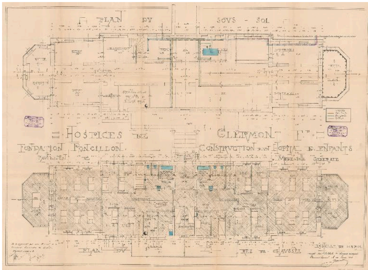
Hôtel-Dieu de Clermont-Ferrand. Le pavillon des militaires et l'hôpital pour enfants, plan du pavillon de médecine générale de l'hôpital pour enfants, 25 février 1913, Jean Amadon, architecte des hospices.
