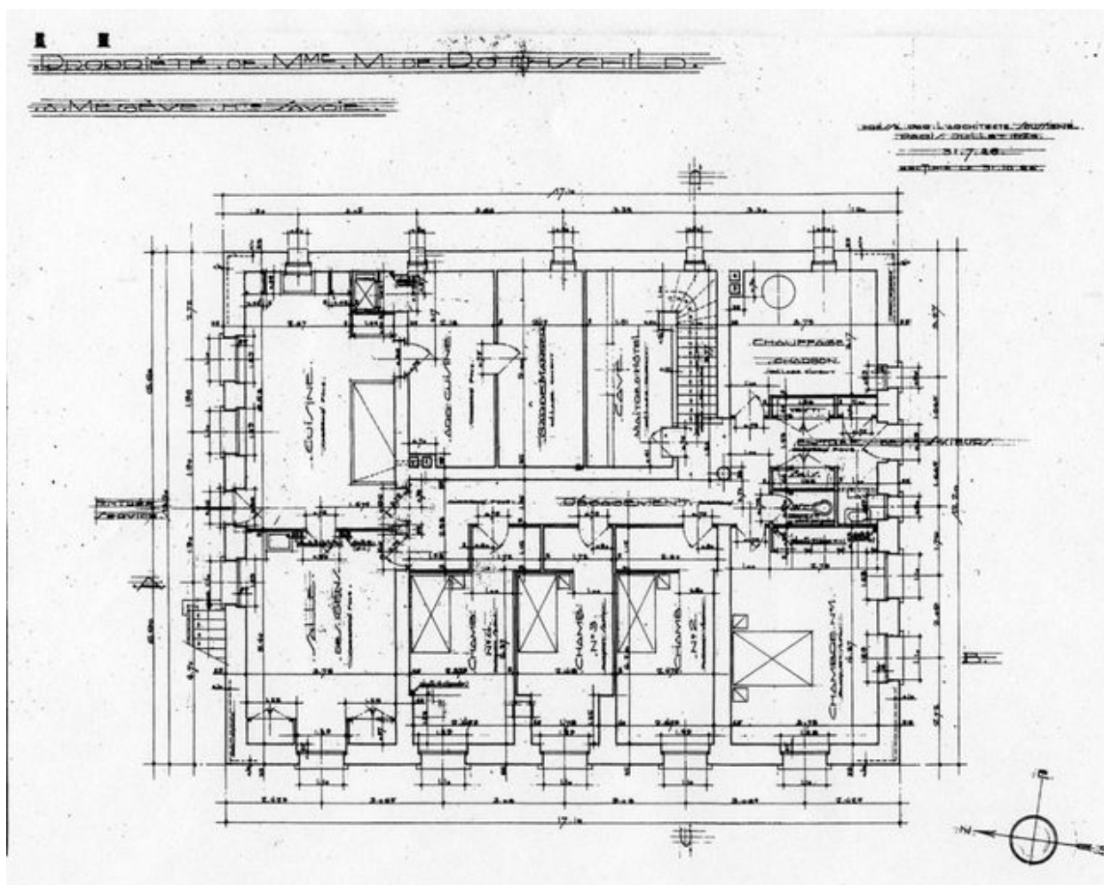
Plan de l'étage de soubassement. Henri Jacques Le Même, 31 juillet 1926. Rectifié le 31 octobre
