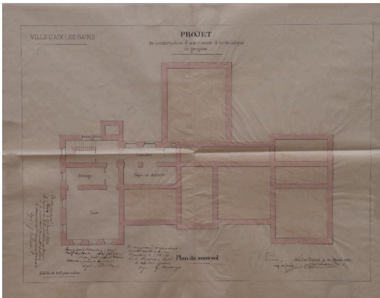
Plan du sous-sol, 1881
