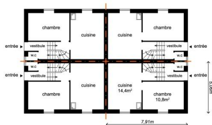
Plan de l'étage des types B ou B'
