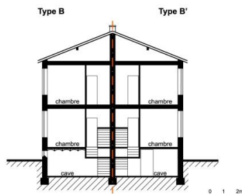
Coupe transversale
