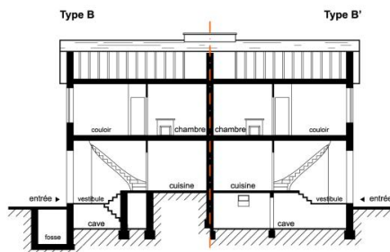
Coupe longitudinale
