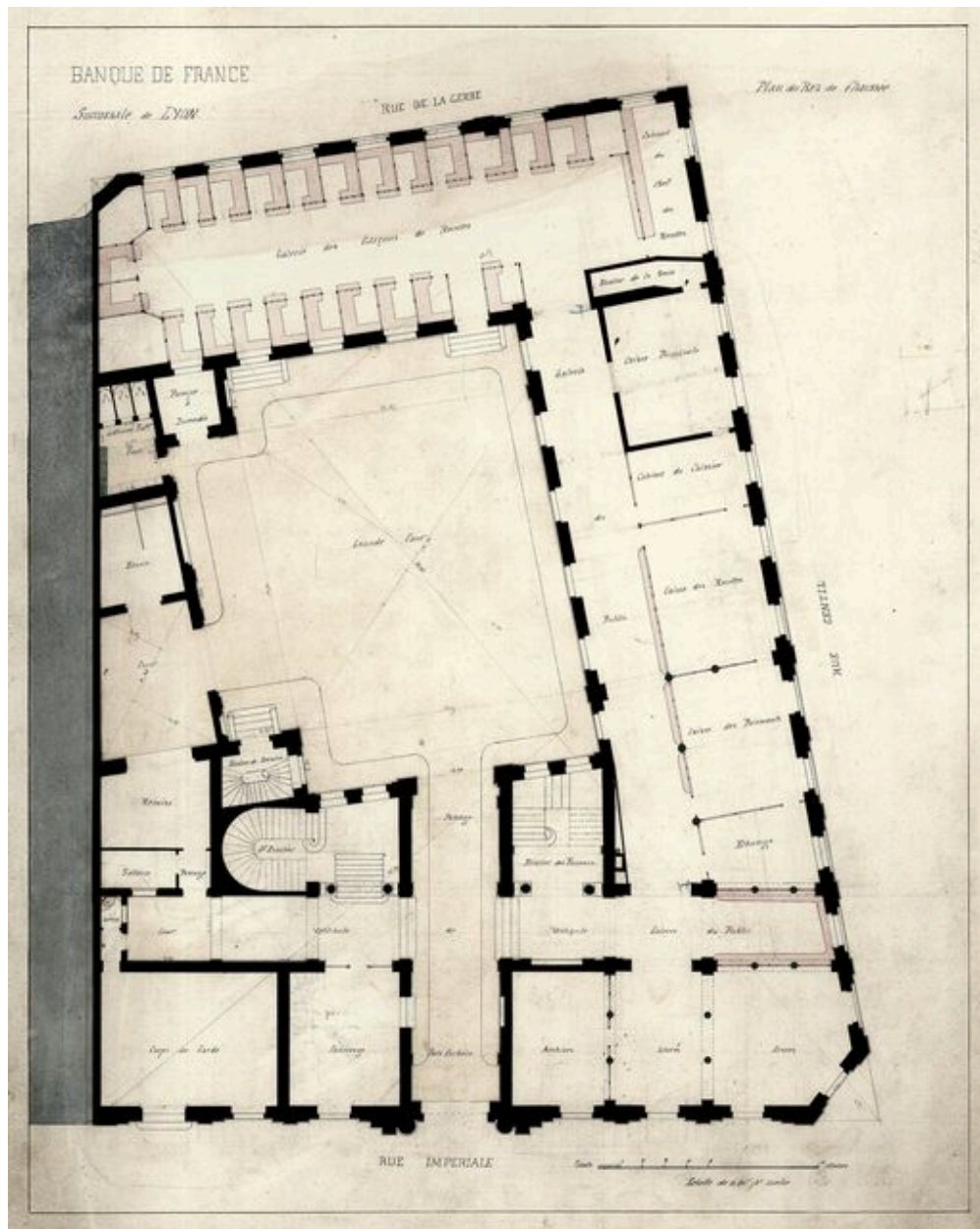
Plan du rez-de-chaussée (vers 1855) (Banque de France, service du Patrimoine Historique et Artistique, non coté, dessin de Gabriel Crétin).
