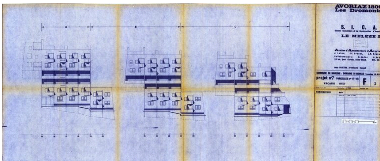
Les Mèlèzes 2. Projet de 1967. Façade sud / J. Labro, J.J. Orzoni, J.M. Roques, 3 janvier 1967 (AC Morzine)
