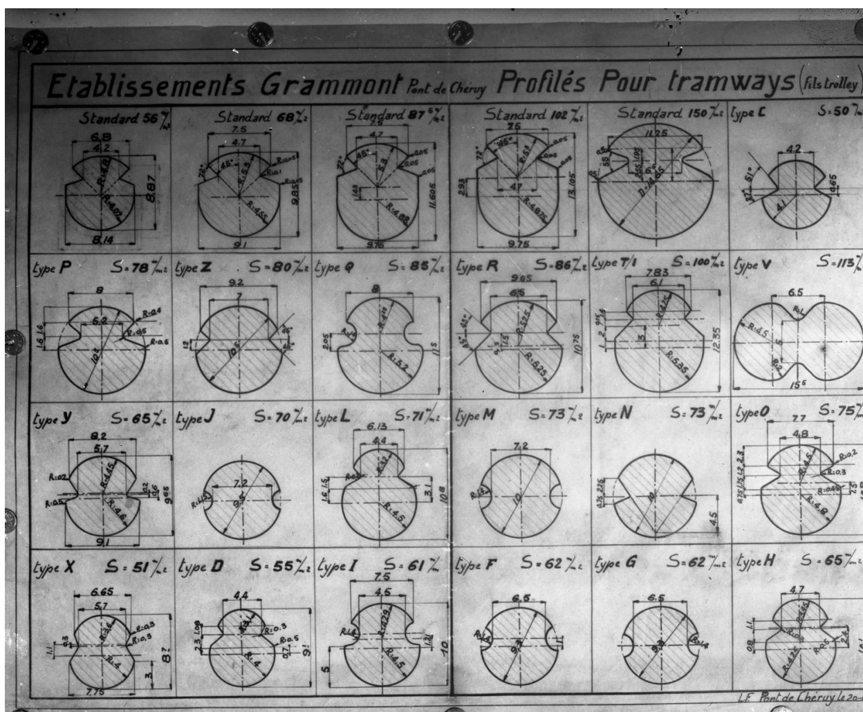
Planche de dessins techniques de profilés pour tramways, AD 69 : série 158 J. usine Tréfimétaux AD Rhône. 158 J
