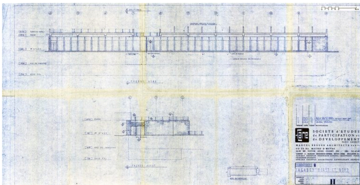
Commerces H. Elévations nord et ouest. Marcel Breuer architecte, 29 novembre 1967 (AC Arâches-la-Frasse)
