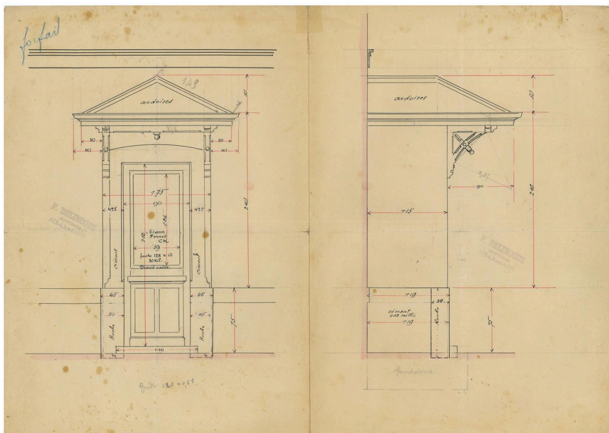
Villa Mireille : plan du porche d'entrée, 1897
