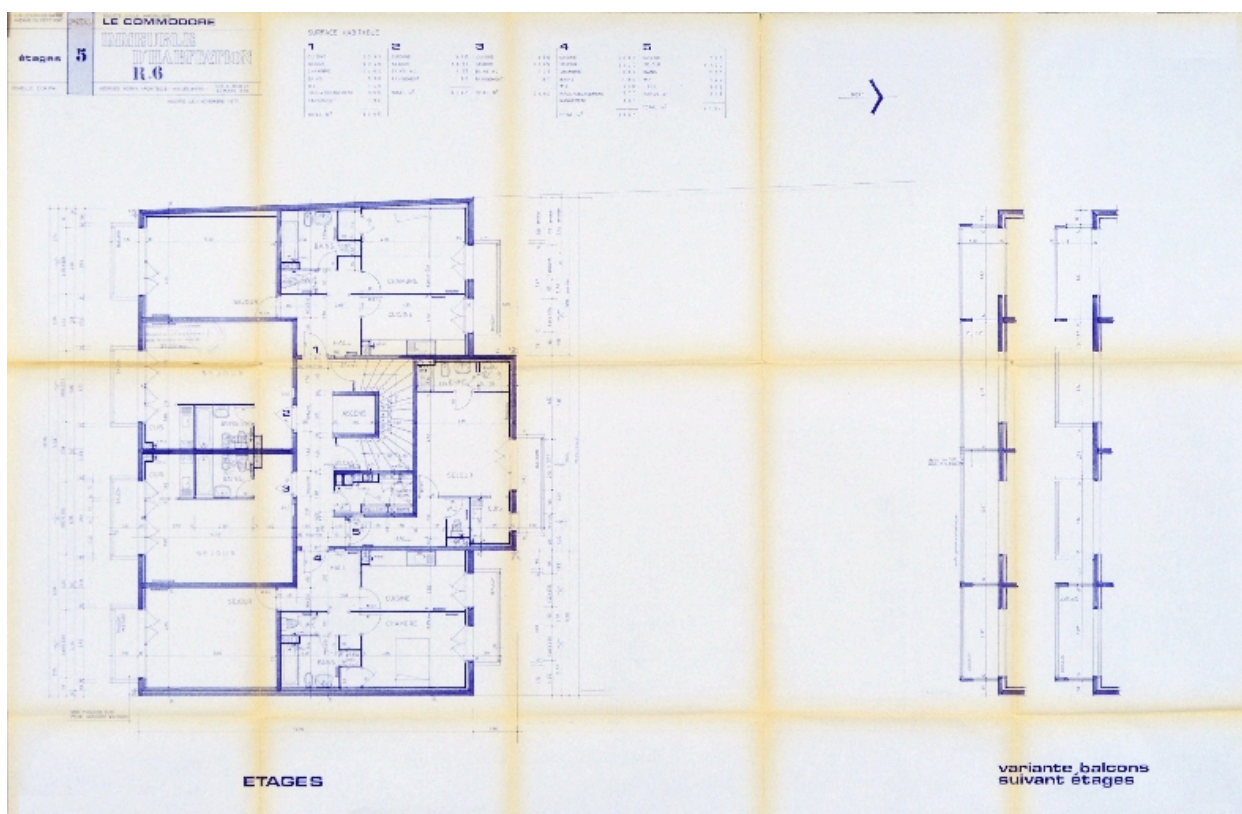
Plan des étages et des balcons
