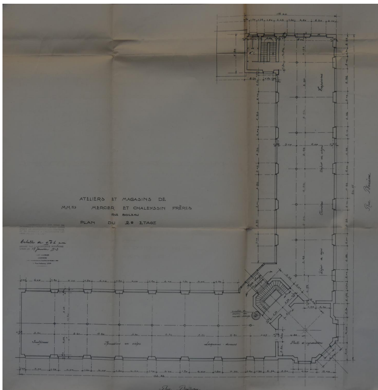
Plan du 2e étage, usine Mercier et Chaleyssin 1913 (ACL 314W515-121)
