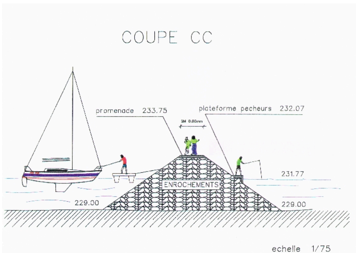
Coupe longitudinale sur l'enrochement, 1991
