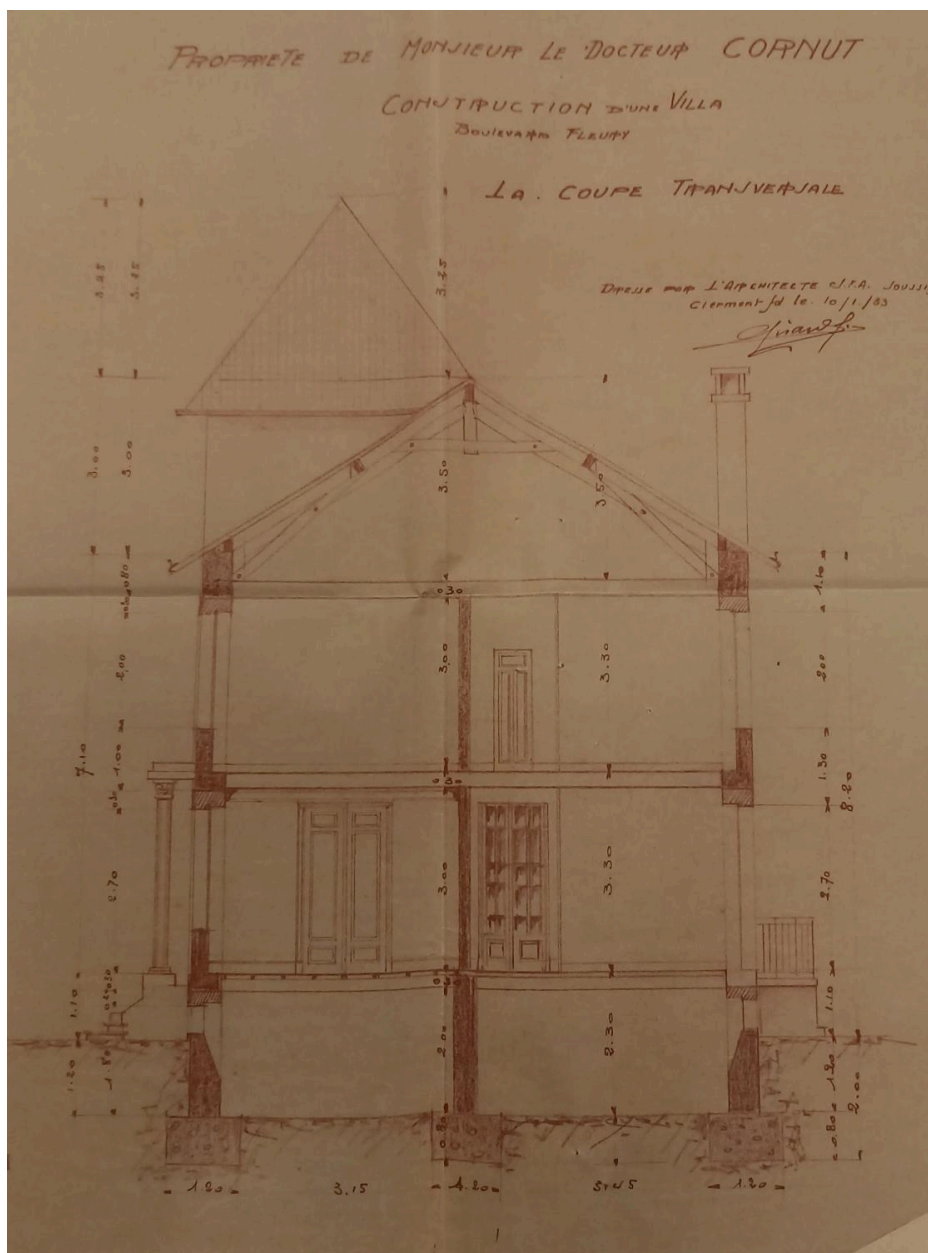
Coupe transversale
