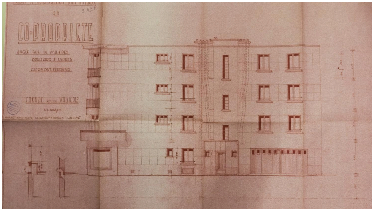
Élévation postérieure sur la rue de Vallières
