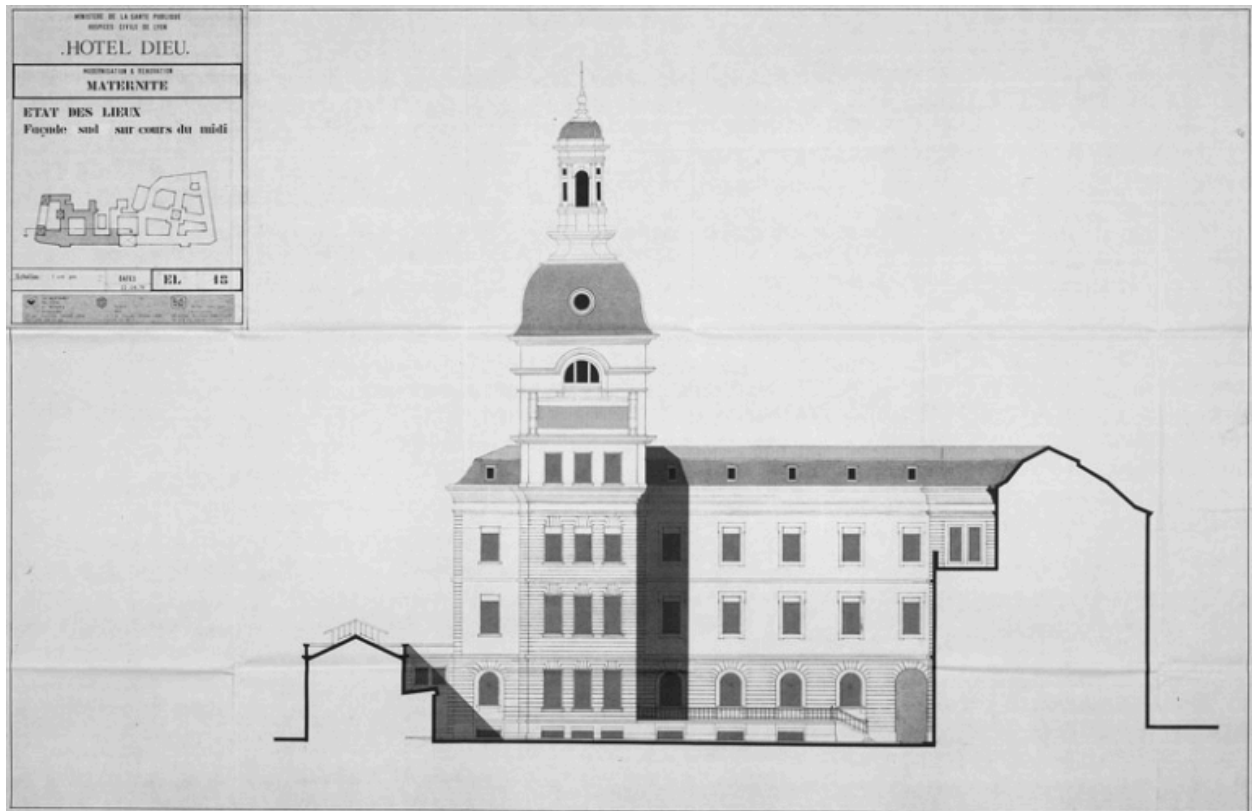
Modernisation et rénovation, maternité. Etat des lieux. Mortamet/Vidal/Manhes. SLETTI. BETSE Caillaud. Facade sud sur la cour du Midi, 22 août 1978
