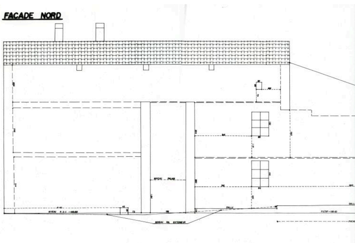
Élévation de la façade nord.
