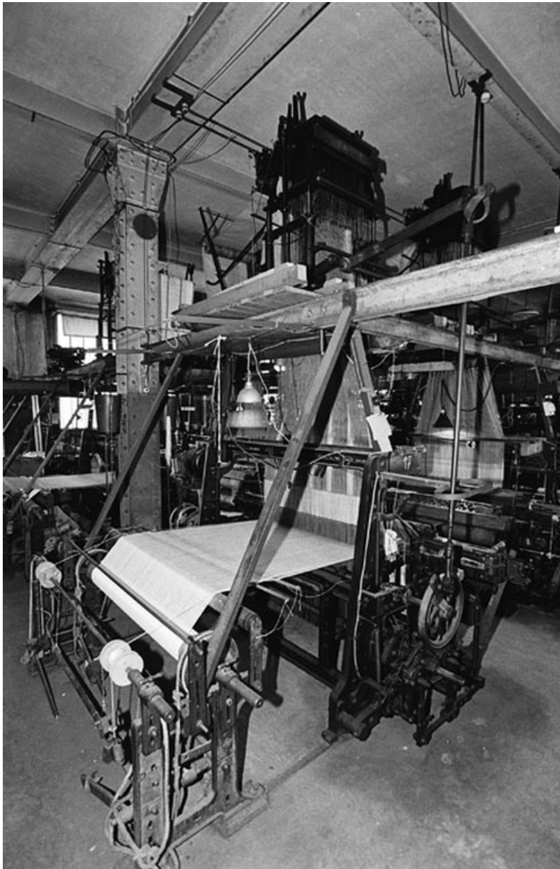
Métier à tisser jacquard n° 17, mécanique Verdol, de marque Diederich
