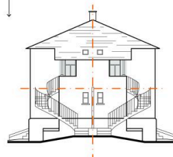
Élévation sur pignon
